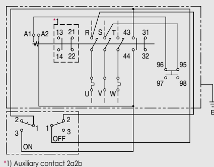
GMW-9B~22B
