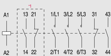
GMC-9~22
